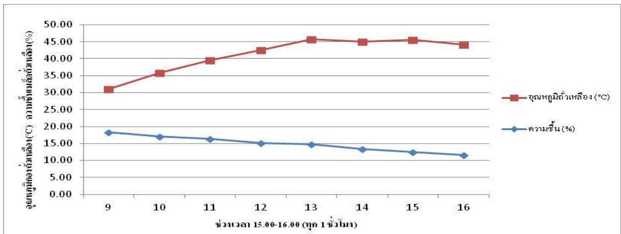
ภาพที่ 5 แสดงอุณหภูมิและความชื้นของเมล็ดถั่วเหลือง ระหว่างการลดความชื้นเมล็ดพันธุ์ถั่วเหลืองด้วยในโรงตากแบบหลังคาทรงโค้ง
