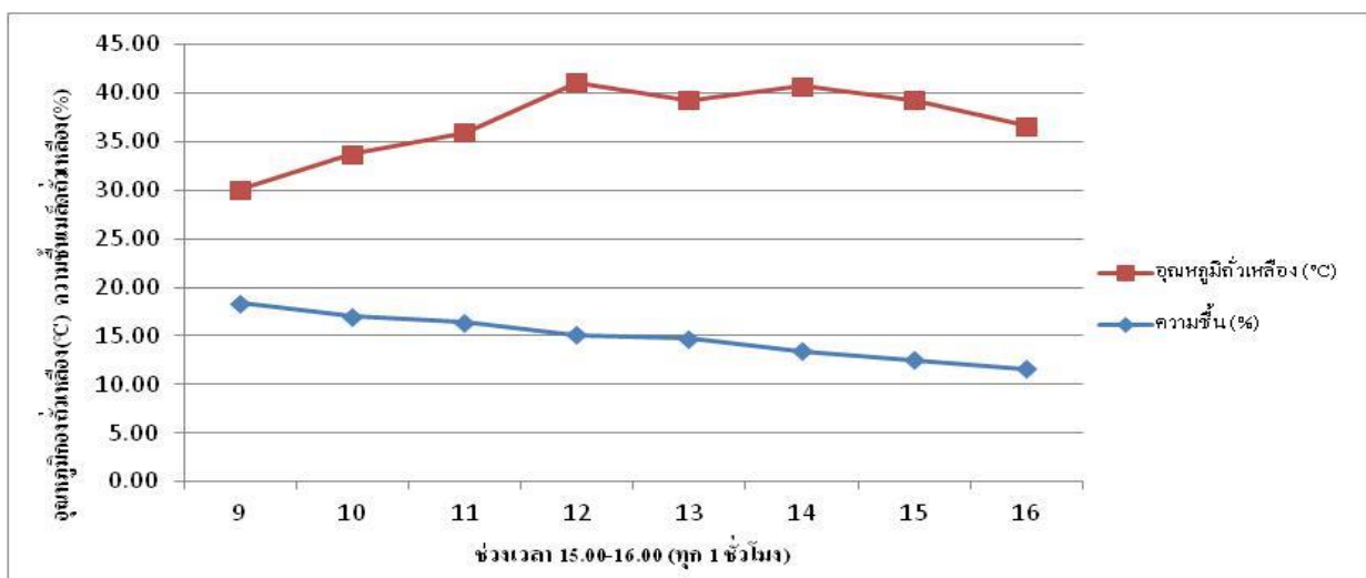
ภาพที่ 6 แสดงอุณหภูมิและความชื้นของเมล็ดถั่วเหลือง ระหว่างการลดความชื้นเมล็ดพันธุ์ถั่วเหลืองด้วยชั้นตะแกรงเหล็ก
