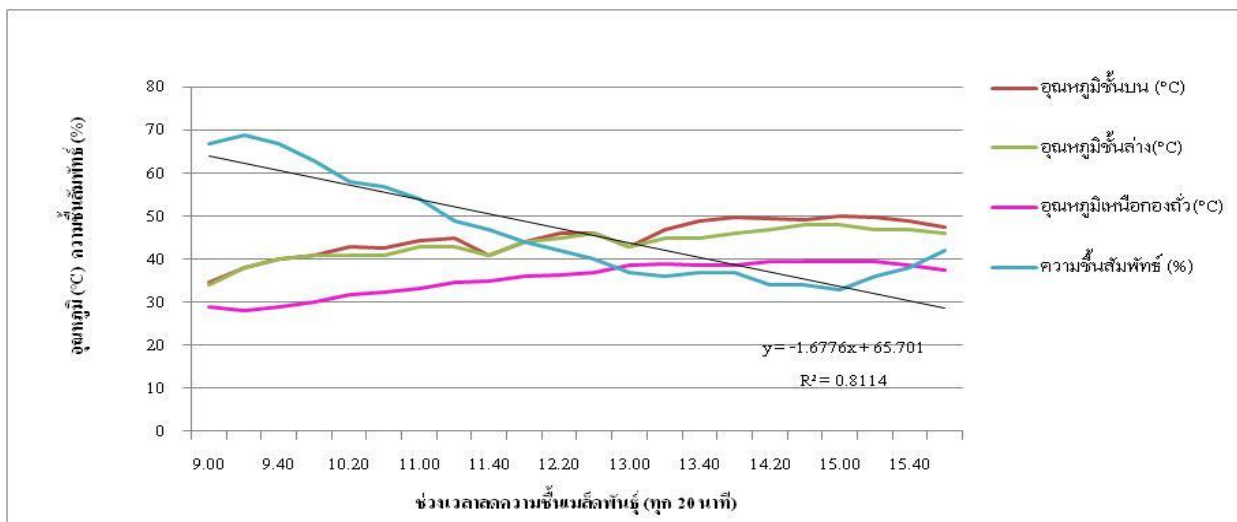
ภาพที่ 9 แสดงอุณหภูมิและความชื้นสัมพัทธ์ภายในโรงตากหลังคาทรงโค้ง ระหว่างการลดความชื้นเมล็ดพันธุ์หัวเลื่อง
