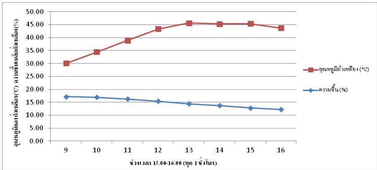
ภาพที่ 4 แสดงอุณหภูมิและความชื้นของเมล็ดถั่วเหลือง ระหว่างการลดความชื้นเมล็ดพันธุ์ถั่วเหลืองด้วยในโรงตากแบบหลังคาน้ำจั่ว
