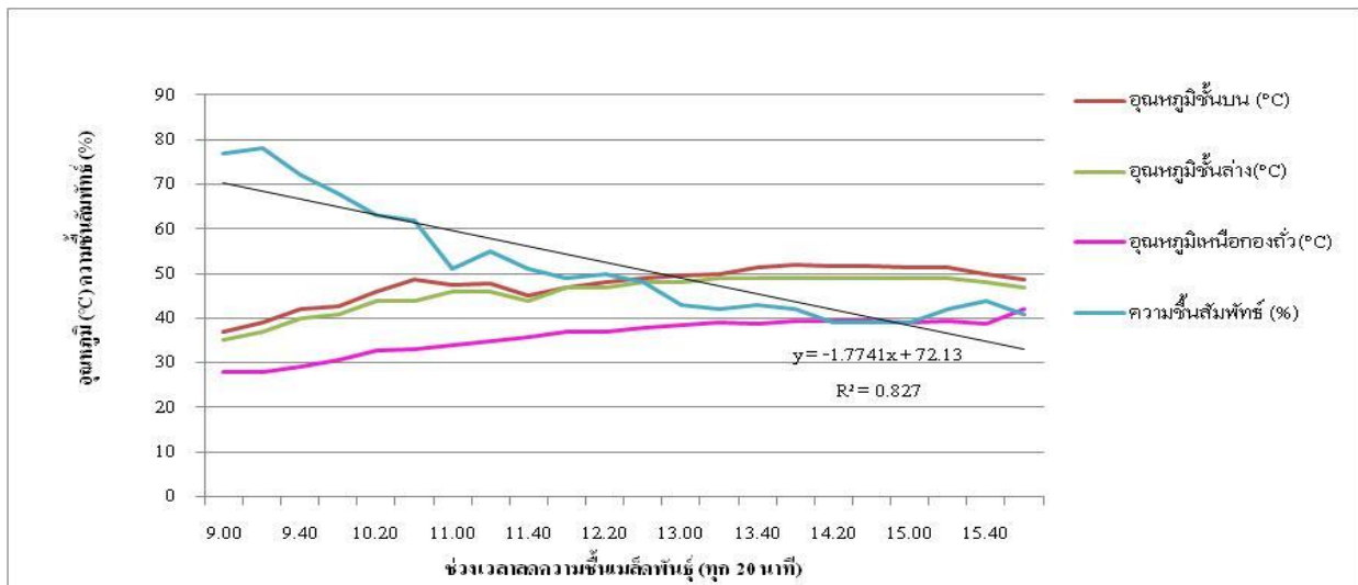
ภาพที่ 8 แสดงอุณหภูมิและความชื้นสัมพัทธ์ภายในโรงตากหลังคาทรงหน้าจั่ว ระหว่างการลดความชื้นเมล็ดพันธุ์หัวเลื่อง
