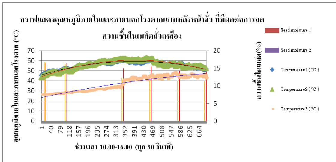
ภาพที่ 1 แสดงอุณหภูมิภายในและภายนอกโรงตากแบบหลังคาหน้าจั่ว ที่มีผลต่อการลดความชื้นในเมล็ดถั่วเหลือง
