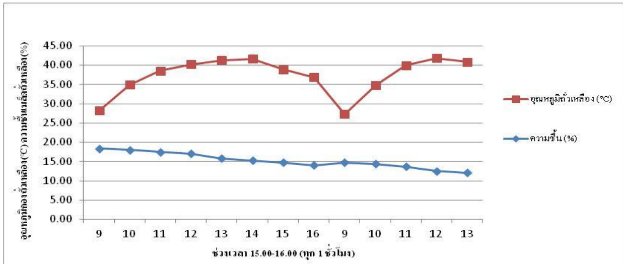
ภาพที่ 7 แสดงอุณหภูมิและความชื้นของเมล็ดหัวเลื่อง ระหว่างการลดความชื้นเมล็ดพันธุ์หัวเลื่องด้วยการตากบนพื้นปูนซีเมนต์
